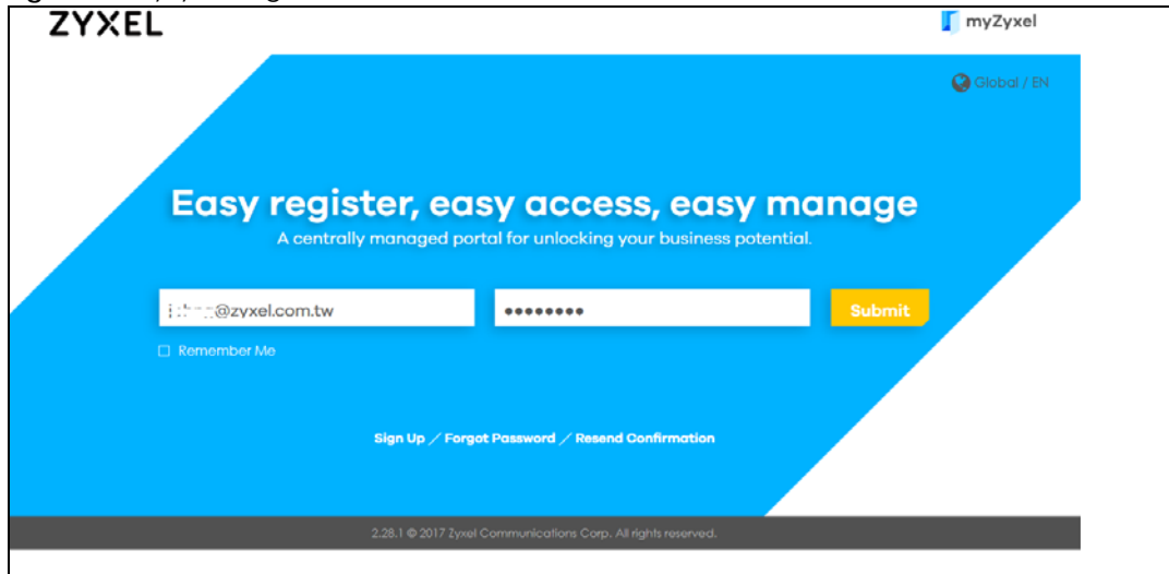
Figure 3 myZyxel Login
