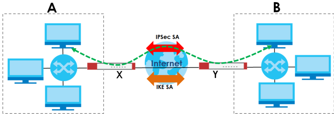
Figure 353 VPN: IKE SA and IPsec SA
