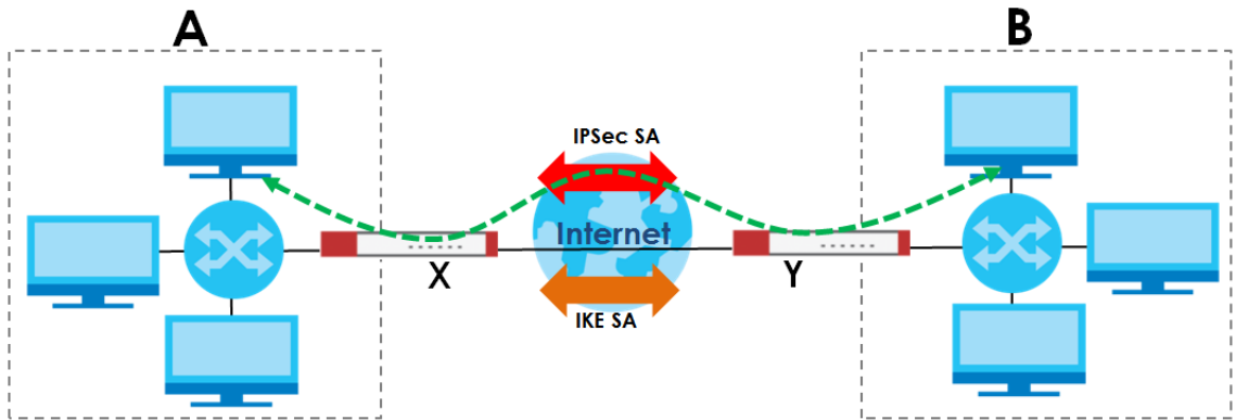
Figure 351 VPN: IKE SA and IPsec SA
