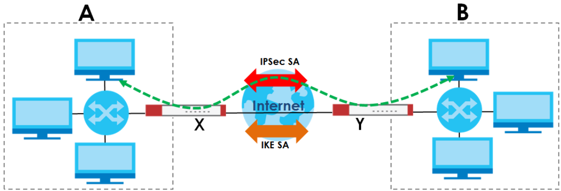
Figure 289 VPN: IKE SA and IPsec SA
