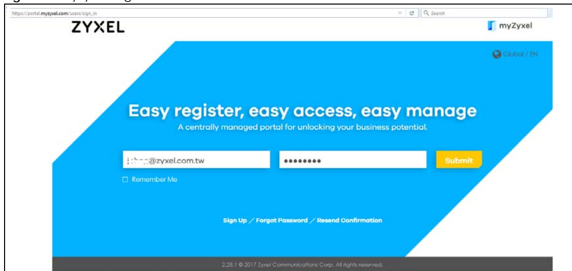
Figure 1 myZyxel Login
