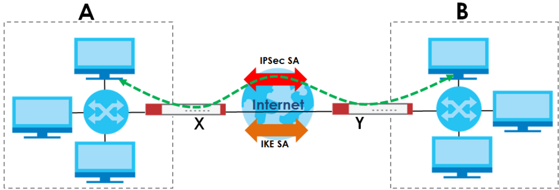
Figure 453 VPN: IKE SA and IPsec SA
