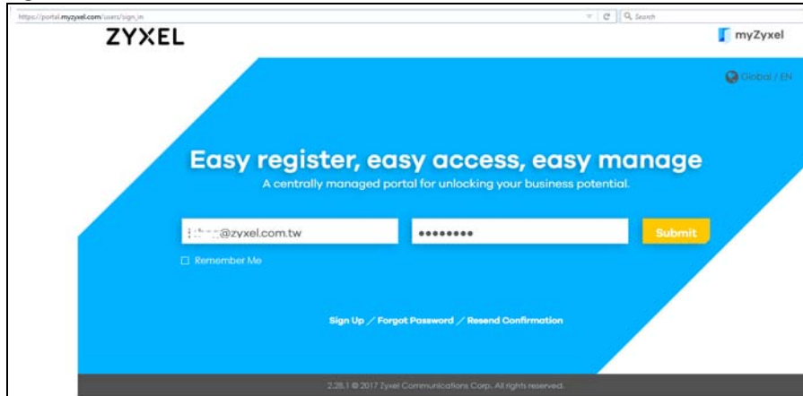
Figure 34 myZyxel Login
